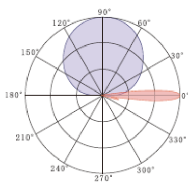
2400MHz
